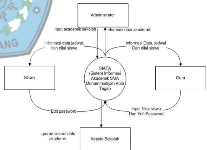
Gambar 3.2 DFD Level 0 (Diagram Konteks SIATA)
