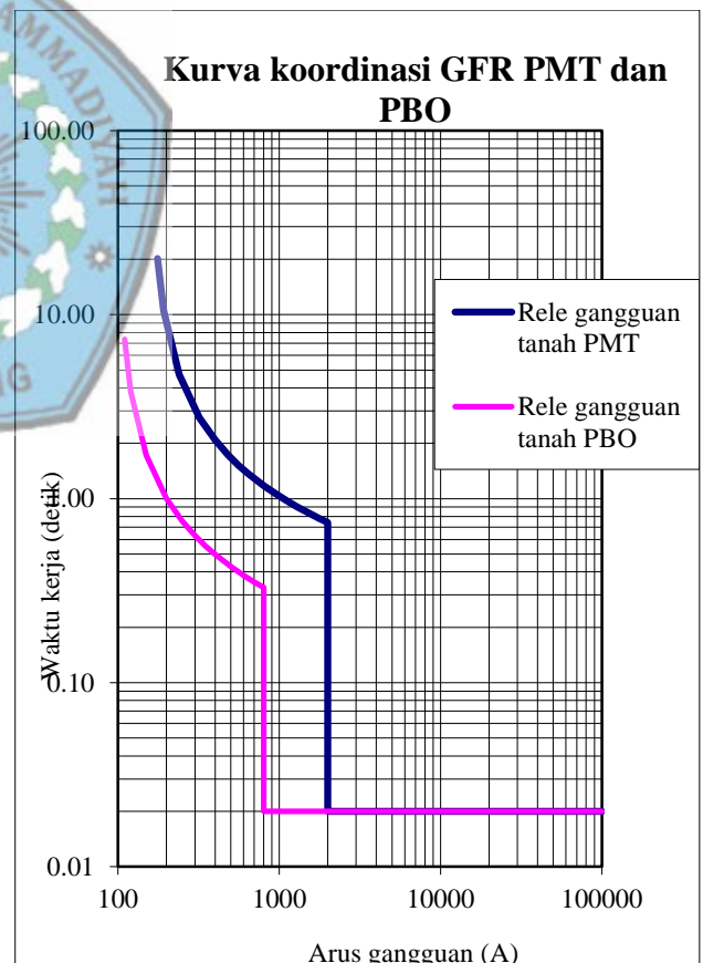
Gambar 3 Kurva koordinasi karakteristik kerja GFR dari PMT dan PBO
