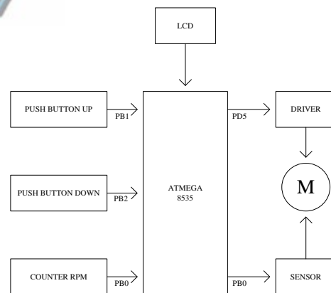
Gambar 3.2. Blok Diagram Sistem Keseluruhan
