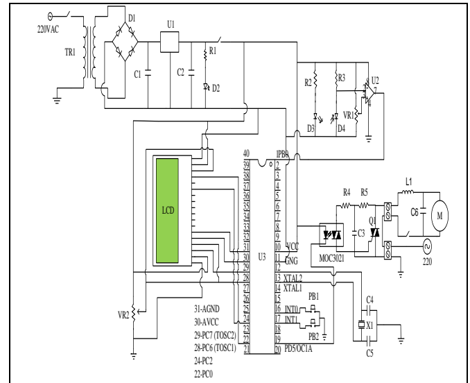
Gambar 3.1. Rangkaian Keseluruhan
