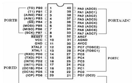
Gambar 2.1. Konfigurasi Pin Microcontroller AVR ATmega8535
