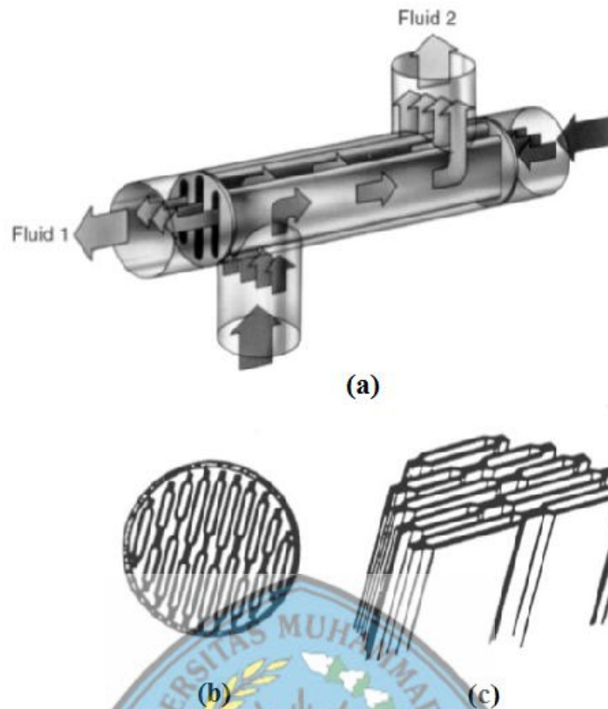
Gambar 2 8. Lamella Heat Exchanger Beserta Desain Emailnya
