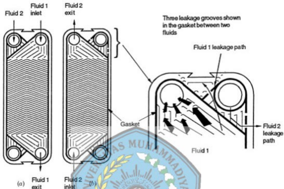
Gambar 2 4. Desain Gasket Untuk Pendistribusian Fluida Kerja
