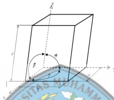
Gambar 2 11. Unit sel dengan koordinat x, y, z panjang sisi a, b, c dan sudut \alpha, \beta, \gamma (Callister,2001)
