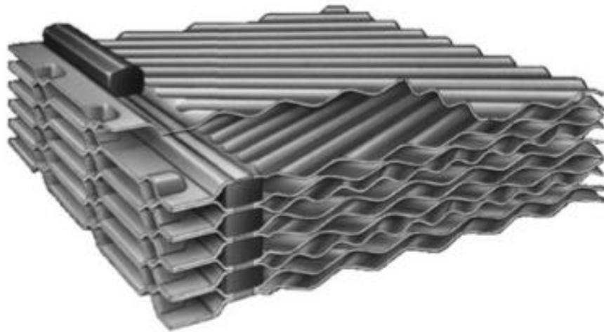
Gambar 2 5. Elemen Plat Pada WPHE
