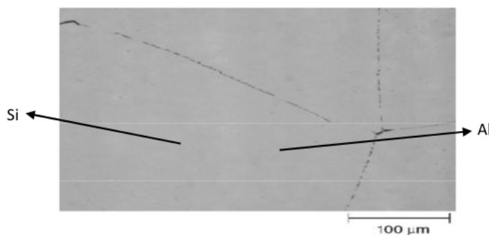
Gambar 3. Struktur Mikro Kawat Aluminium
