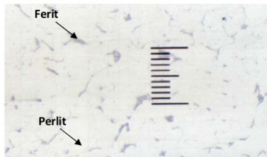
Gambar 4. Struktur Mikro Permukaan Pipa Baja Galvanis
