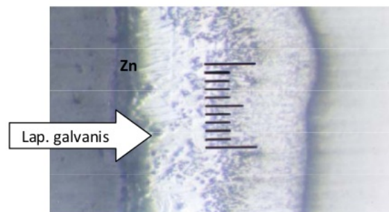
Gambar 5. Struktur Mikro Lapisan Galvanis Bagian Dalam Pipa
