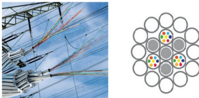
Gambar 2. Susunan Kabel OPPC
