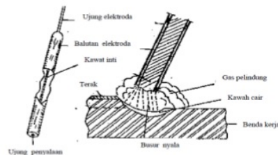
Gambar 3. Kawat elektroda
