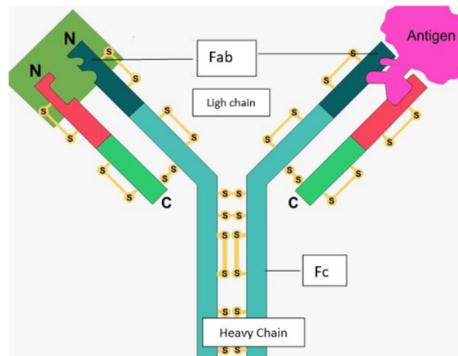
Gambar 5. Struktur antibody
