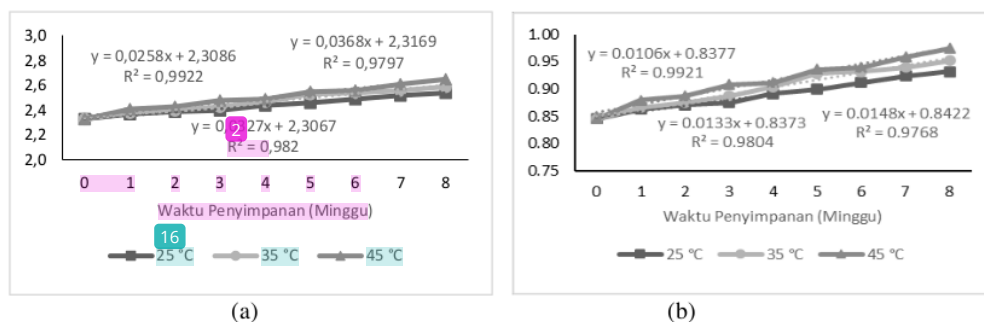
Gambar 1 Persamaan regresi linear kadar air pada (a) ordo 0 dan (b) ordo 1
