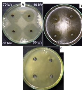
Gambar 1. (A: konsentrasi ekstrak sirih merah 40, 50, 60, dan 70% b/v, B: Kontrol Positif Fluconazole 10 \mu\text{g/mL} , C: Kontrol Negatif DMSO).
