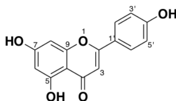
Gambar 1. Struktur apigenin (1)
