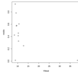
Gambar 3 Plot nilai Y fit dan Nilai Residual
