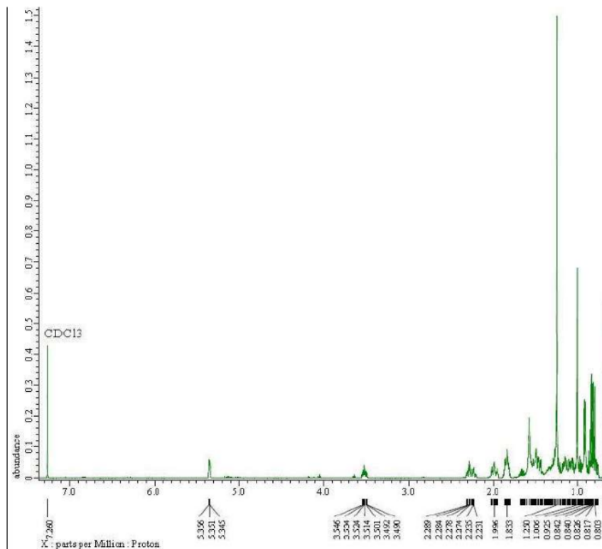
Gambar 2. Spektrum ^1\text{H NMR} Isolat 1.
