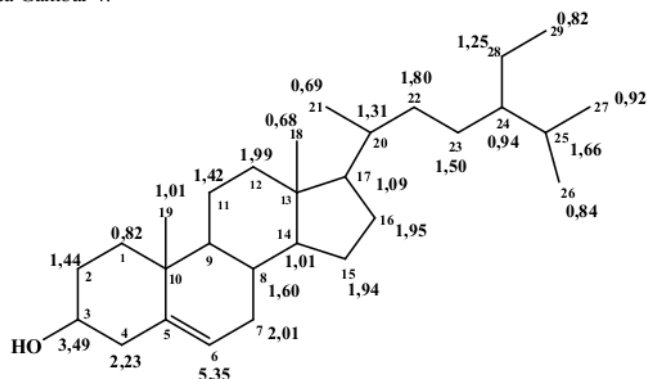
Gambar 4. Struktur stigmaster-5-en-3 \beta -ol ( \beta -sitosterol).
