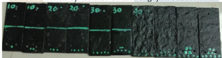
Gambar 2 Bahan Uji Isolator Untuk Pengujian Sudut Kontak
