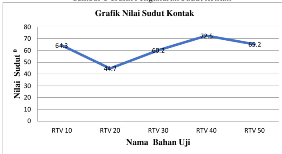
Gambar 3 Grafik Pengukuran Sudut Kontak
