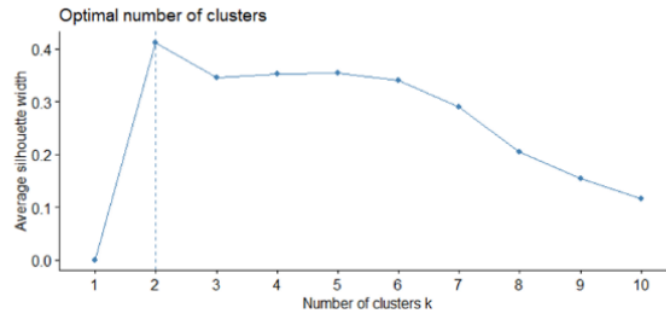
Gambar 1. Grafik Elbow
