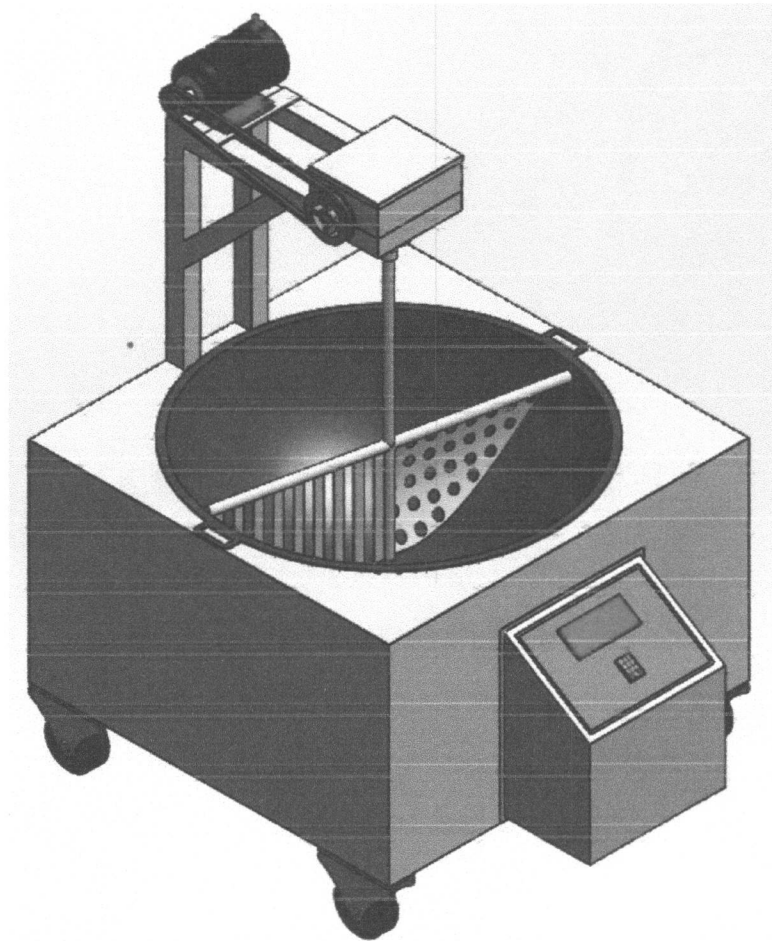
Gambar 1. Desain tiga dimensi alat pengolah Gula Semut
